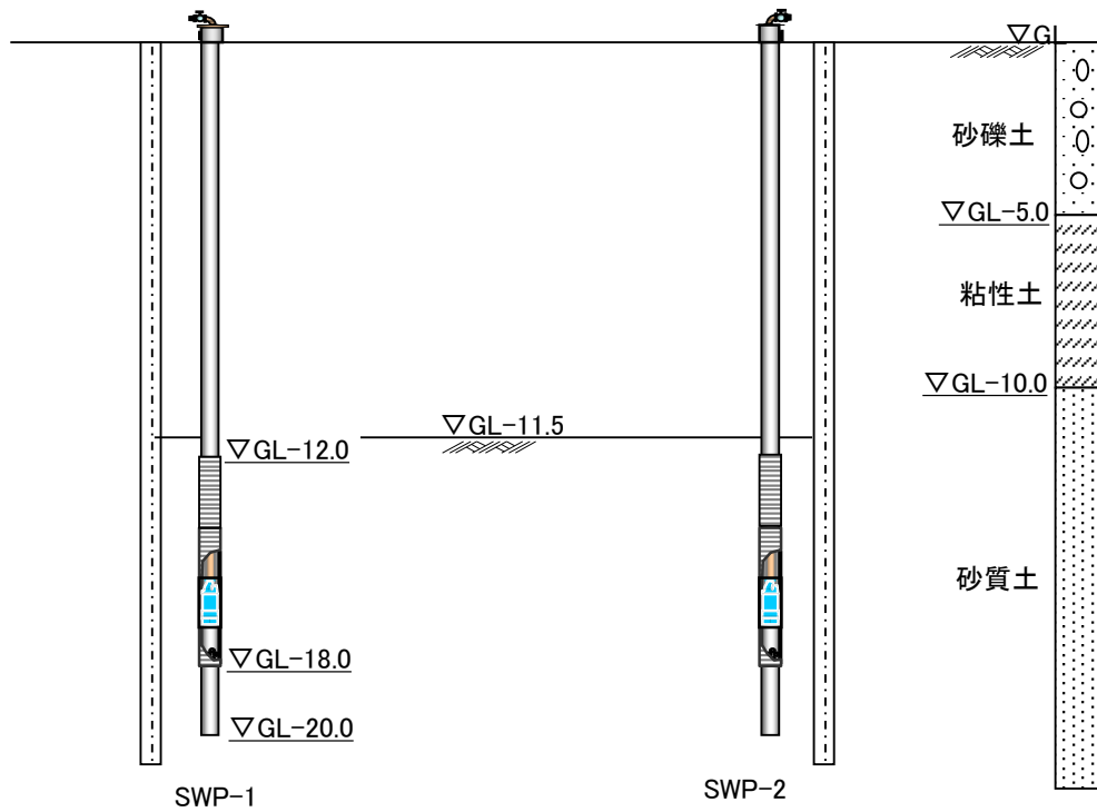
断面図
