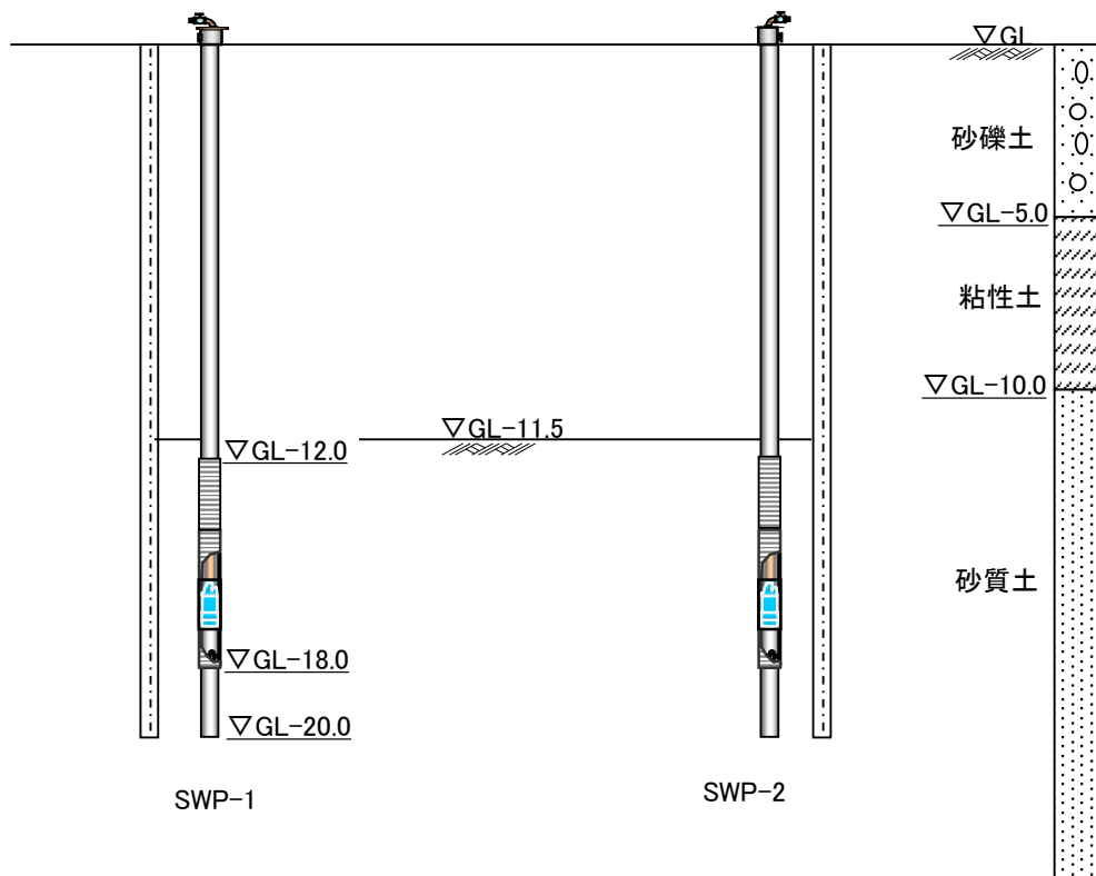
断面図
